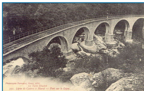
Le viaduc des Labans lors de sa construction en 1906
